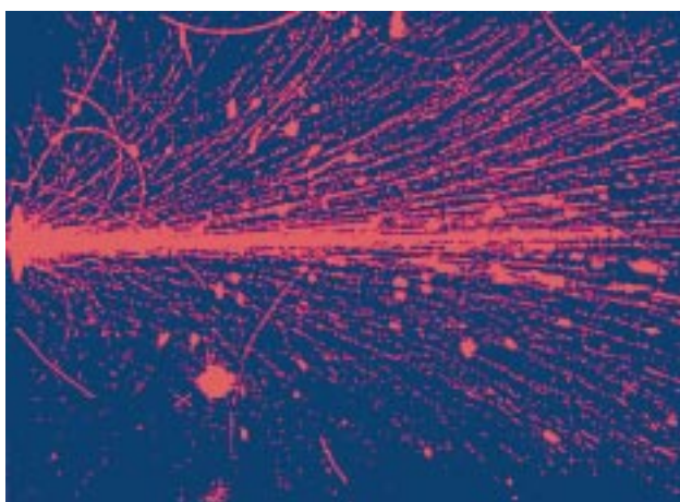
Рис. 3. Фотография столкновения ядер S и Au в стримерной камере
