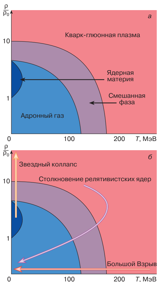
Рис. 1. а – фазовая диаграмма адронной материи; б – различные физические процессы на фазовой диаграмме
