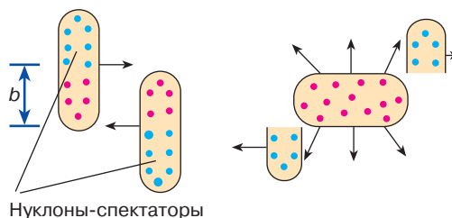
Рис. 4. Геометрия столкновений ядер с прицельным параметром b
